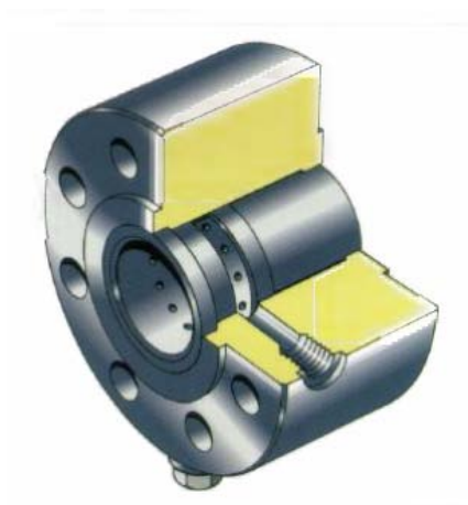
Fig D.1 BV986 Mini Desuperheater
